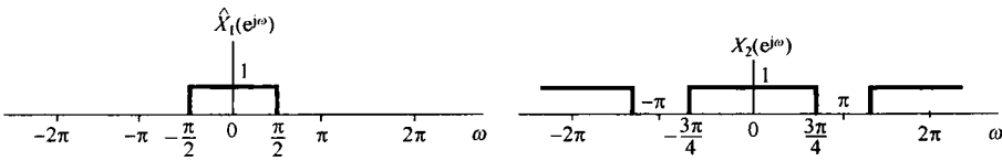
图 5.19 代表 X_1(e^{j\omega}) 的一个周期的 \hat{X}_1(e^{j\omega}) 及 X_2(e^{j\omega}) 。 \hat{X}_1(e^{j\omega}) 和 X_2(e^{j\omega}) 的线性卷积就相应于 X_1(e^{j\omega}) 和 X_2(e^{j\omega}) 的周期卷积
