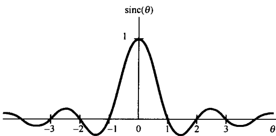
图 4.10 sinc 函数
